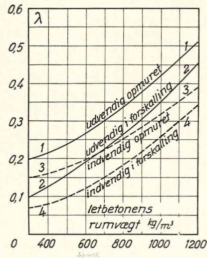
Fig. 3. Varmeledningstal for letbeton i blokke eller plader.
